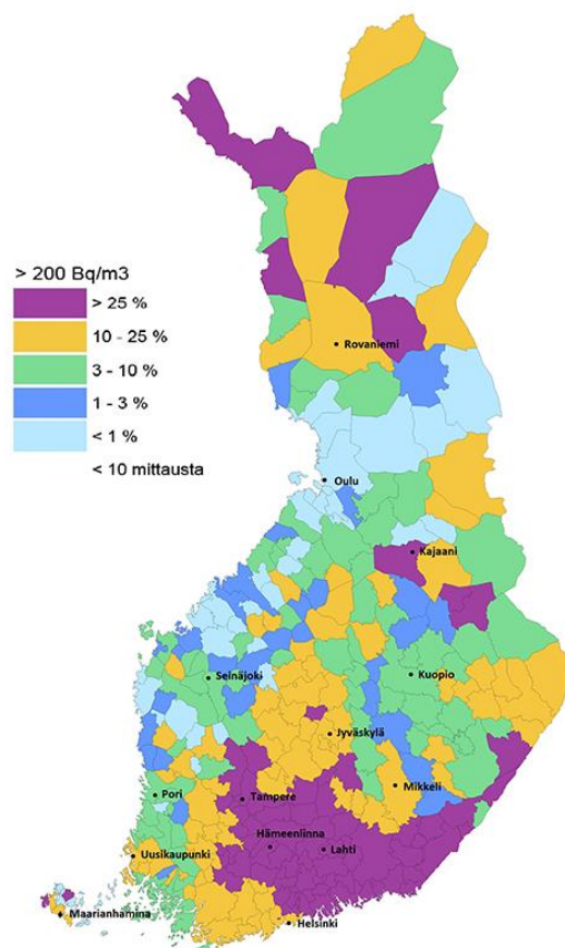
Bild 9. Radon i kommunerna i Finland år 2017 Strålsäkerhetscentralen, www.stuk.fi
